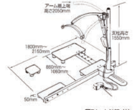
■Bセット外観寸法
