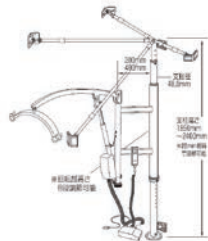
■F2RSKKセット外観寸法
